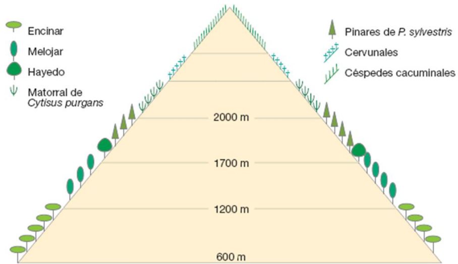
ESQUEMA DE LA CLISERIE ALTITUDINAL DE LA VEGETACIÓN DE LA SIERRA DE GUADARRAMA (Simplificado. Tomado de Bellot)
